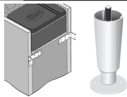
Befestigungswinkel Marine-Fuß
